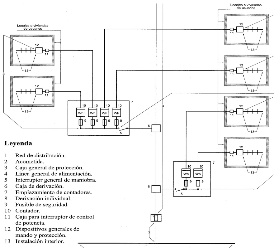
Esquema 2.2.3. Para varios usuarios con contadores en forma centralizada en más de un lugar
