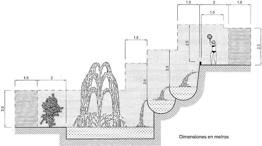
Figura 5. Volúmenes de protección en fuentes
