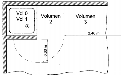
Figura 4. Ducha con pared fija
