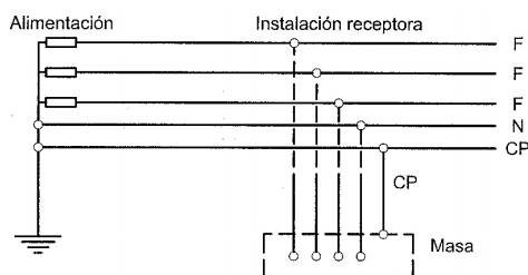
Figura 1. Esquema de distribución tipo TN-S
