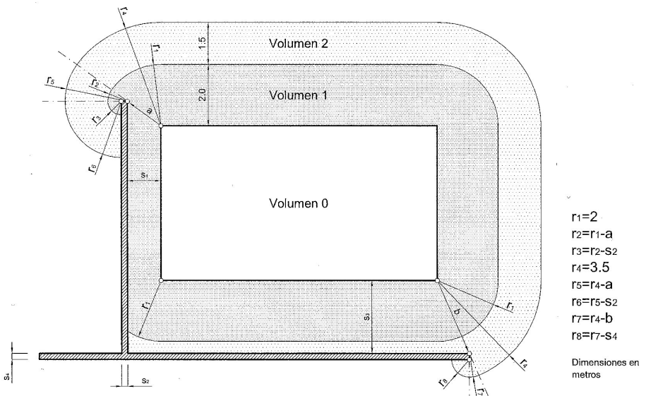
Figura 4. Volúmenes de protección en piscinas con paredes
