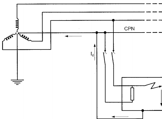
Figura 2. Esquema TN-C
