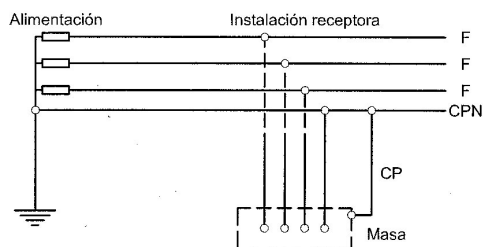
Figura 2. Esquema de distribución tipo TN-C
