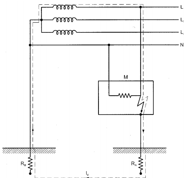
Figura 4. Esquema TT
