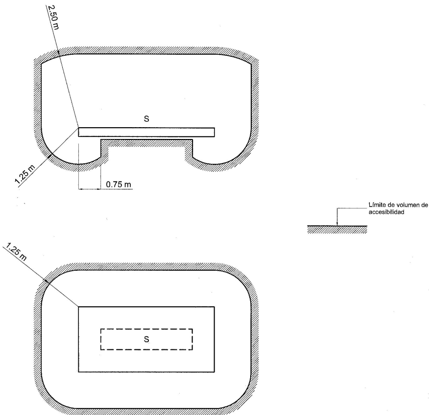
Figura 1. Volumen de accesibilidad
