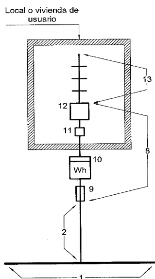
Esquema 2.1. Para un solo usuario
