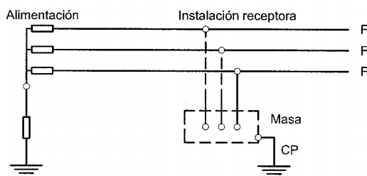
Figura 5. Esquema de distribución tipo IT
