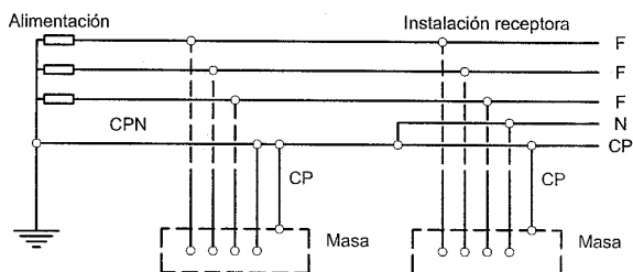
Figura 3. Esquema de distribución tipo TN-C-S
