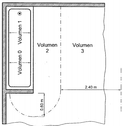
Figura 2. Bañera con pared fija
