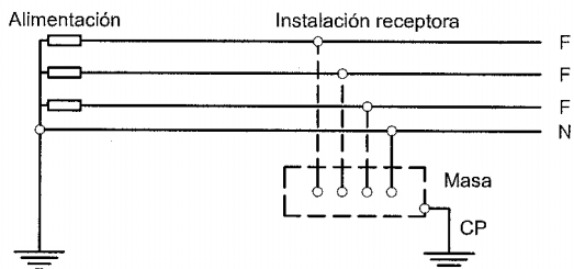
Figura 4. Esquema de distribución tipo TT
